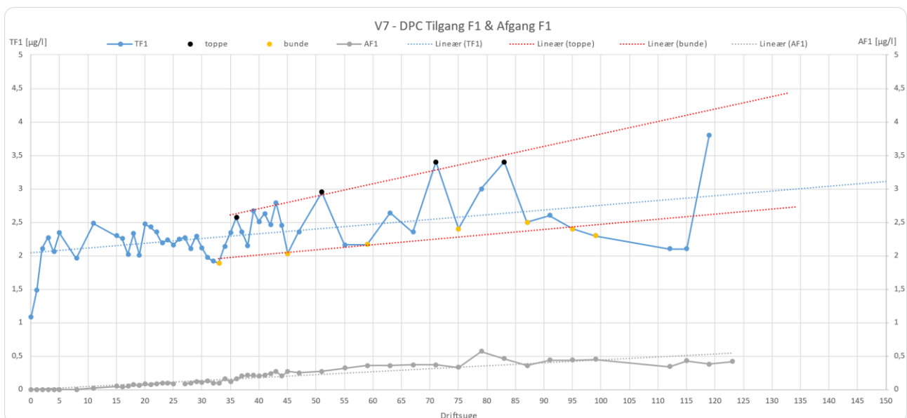
Fig. 1. Grafen viser, at tilgangen til filter 1 stadigvæk stiger (DPC) og afgang fra filter 2 viser en rensning ned til 0,04 mikrogram/liter
